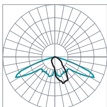
Curva Polar
